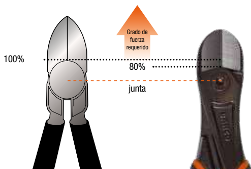
COMPARACIÓN DE PALANCA Cortantes diagonales estándar y cortantes diagonales "heavy duty"
